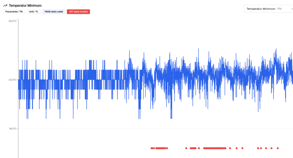
Gambar 4.9. Visualisasi Time-Series
